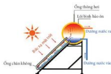
▲ Hình 8.8. Nguyên lý hoạt động của máy nước nóng năng lượng mặt trời
