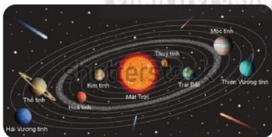
▲ Hình 5.14. Minh họa hệ Mặt Trời
