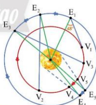
Hình 5.17. Vị trí của Trái Đất (E) và Kim tinh (V) quan Mặt Trời tại một số thời điểm
