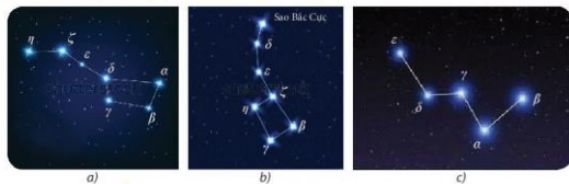
▲ Hình 4.4. Ba chòm sao: a) Gấu Lớn; b) Gấu Nhỏ; c) Thiên Hậu
