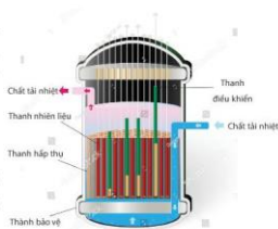
▲ Hình 2.1. Lò phản ứng hạt nhân
