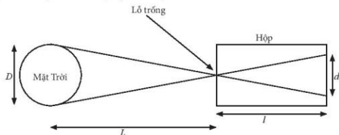
▲ Hình 6P.3. Mô hình đơn giản Aristarchus sử dụng để đo đường kính của Mặt Trời
