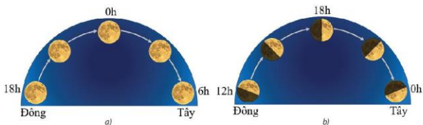
▲ Hình 5.4. Hình ảnh quan sát từ mặt đất về đường đi của Mặt Trăng trên bầu trời vào: a) ngày rằm; b) ngày 8 âm lịch hàng tháng
