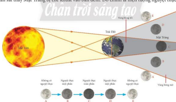
▲ Hình 6.9. Quá trình diễn ra hiện tượng nguyệt thực
