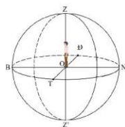
Hình 4.1. Mô hình thiên cầu
