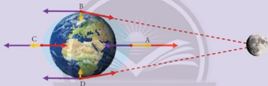
▲ Hình 6.16. Minh họa lực tương tác giữa Mặt Trăng và các khối nước trên bề mặt Trái Đất
