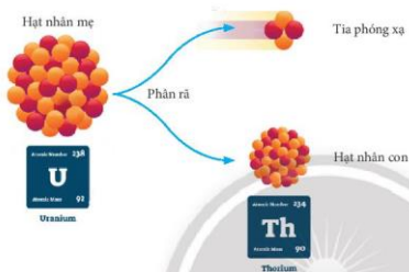
▲ Hình 10.7. Quá trình phân rã phóng xạ
