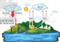
▲ Hình 10.6. Quy trình tạo thành mưa acid
