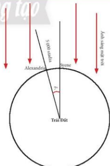
▲ Hình 5.9. Mô hình tính chu vi Trái Đất
