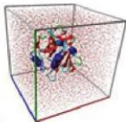
▲ Hình 3.18. Mô phỏng MD để nghiên cứu DNA
